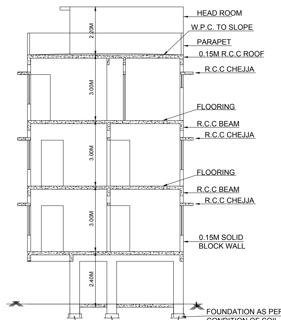
SECTION A-A
